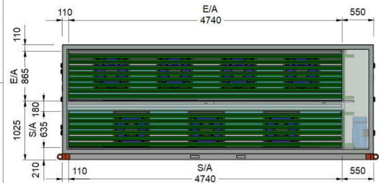
EA & SA SPIGOT VIEW
