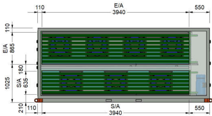
EA & SA SPIGOT VIEW
