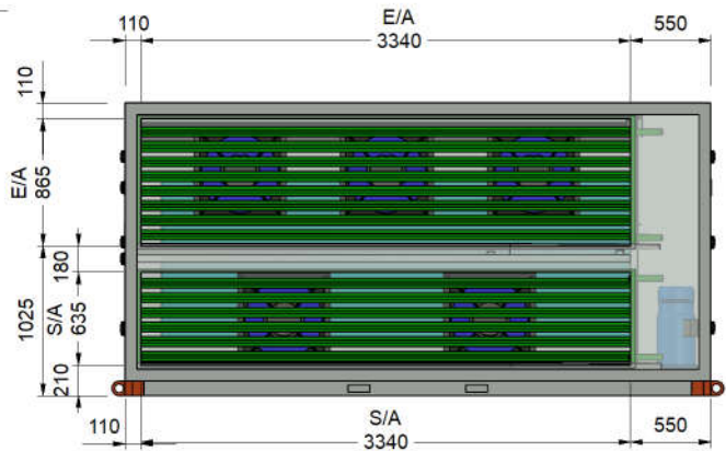
EA & SA SPIGOT VIEW
