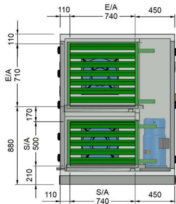
EA & SA SPIGOT VIEW
