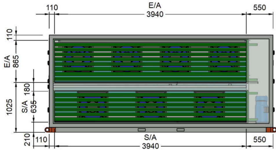
EA & SA SPIGOT VIEW
