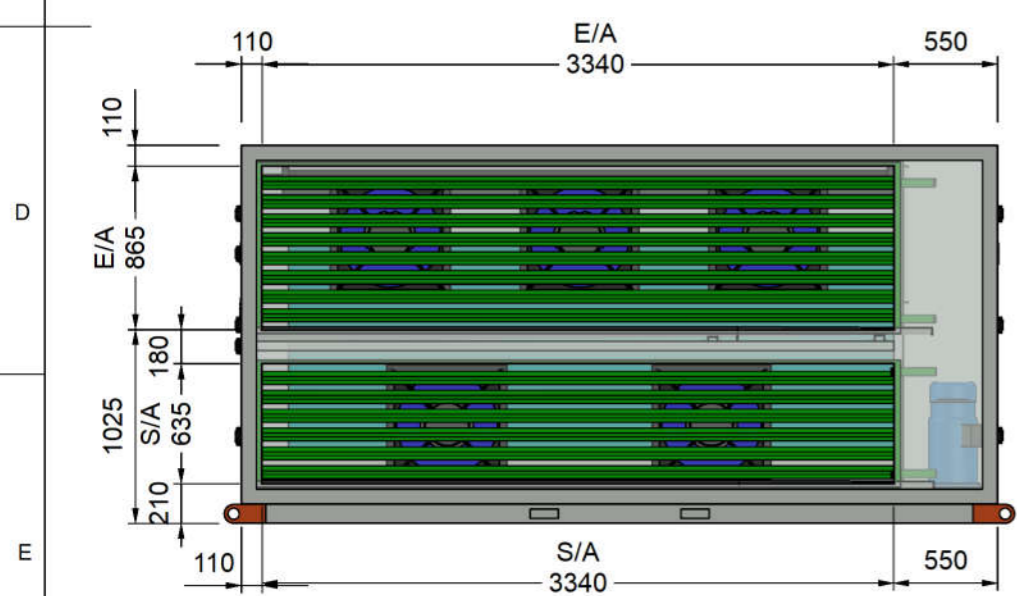
EA & SA SPIGOT VIEW
