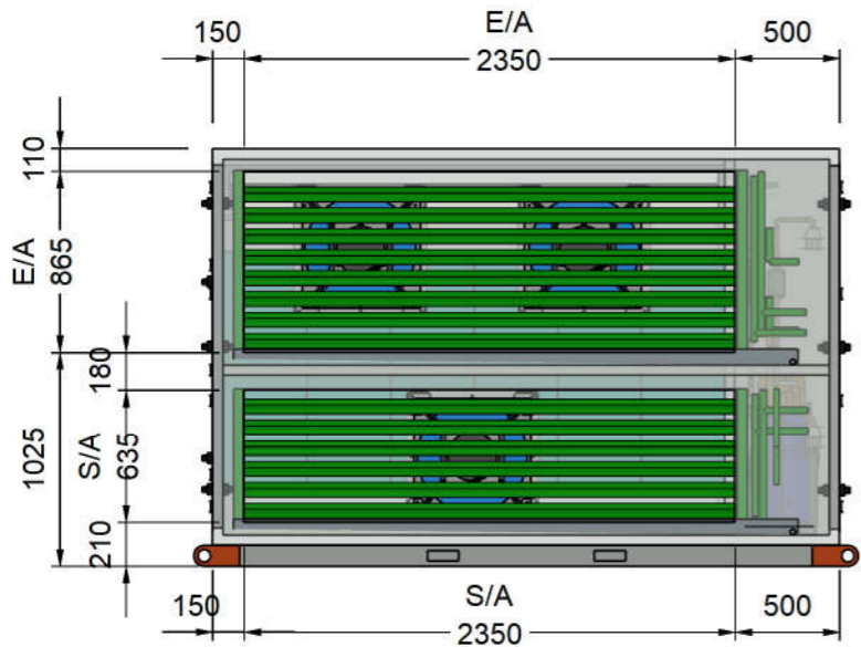
EA & SA SPIGOT VIEW
