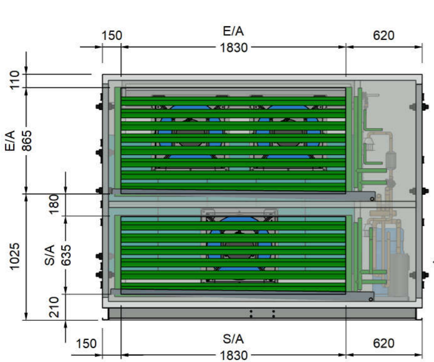
EA & SA SPIGOT VIEW
