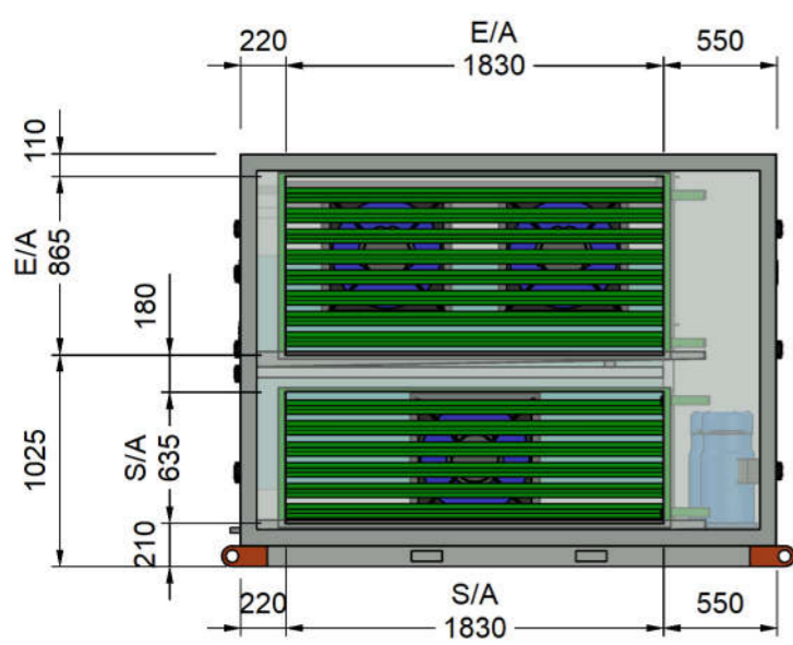
EA & SA SPIGOT VIEW
