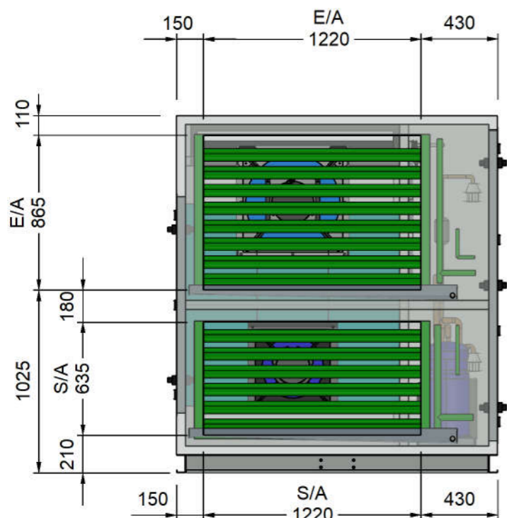
EA & SA SPIGOT VIEW
