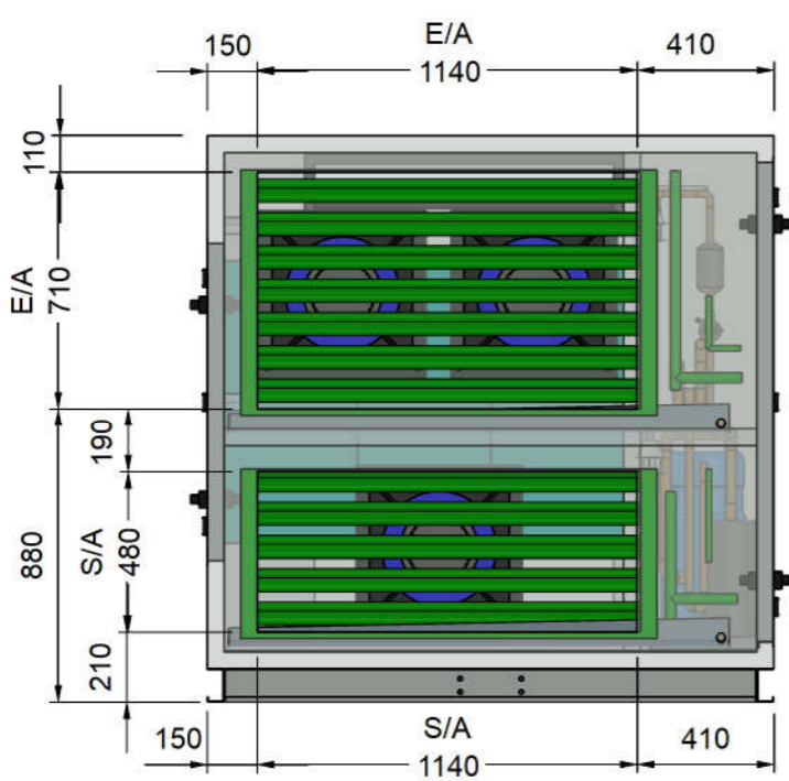
EA & SA SPIGOT VIEW
