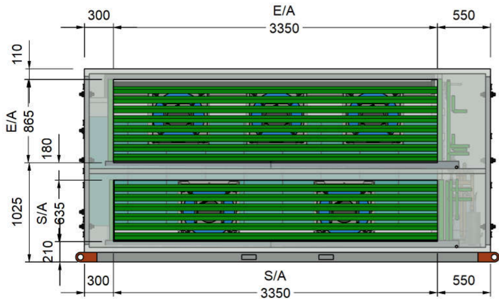
EA & SA SPIGOT VIEW
