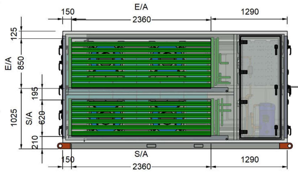
EA & SA SPIGOT VIEW
