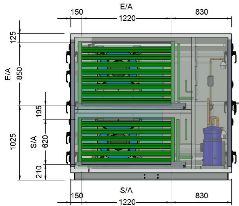
EA & SA SPIGOT VIEW
